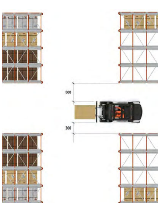
Holguras en pasillos de maniobra Circulación con personal, según UNE-EN 15629
