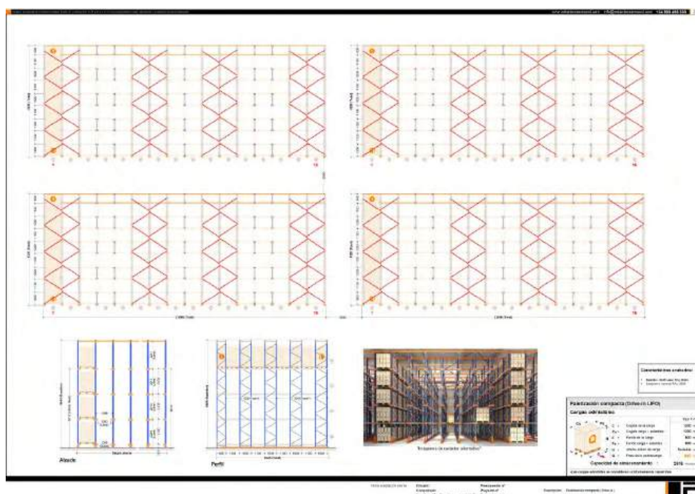
Instalación típica de paletización compacta
