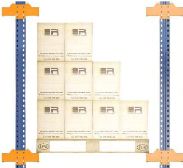
Alzado sobrecarga por asimetría de carga en la paleta Perfil sobrecarga por asimetría de carga en la paleta
