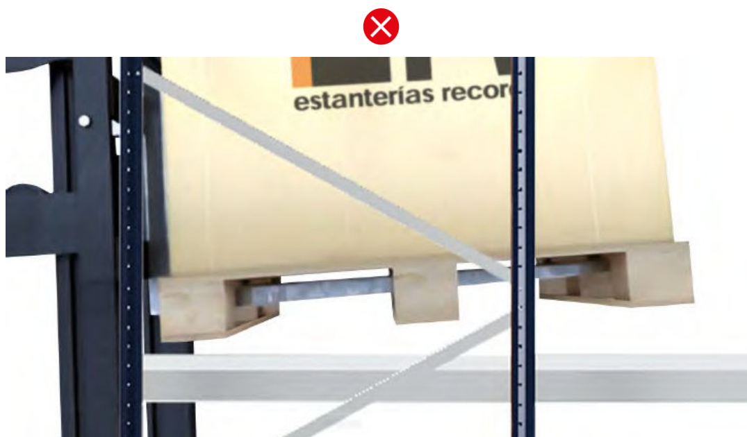
Sobrecargas en carril por descenso no horizontal
