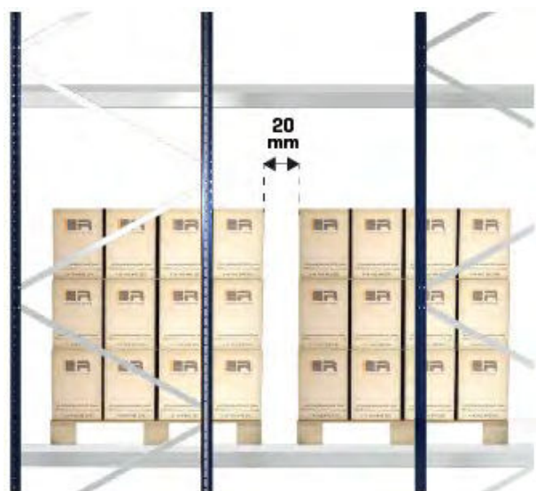
Holguras horizontales en fondo Paletas con carga sin saliente
