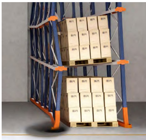
Colapso de la estructura por asentamiento del suelo bajo un bastidor
