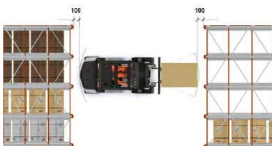
Holguras pasillo de trabajo, circulación simple
