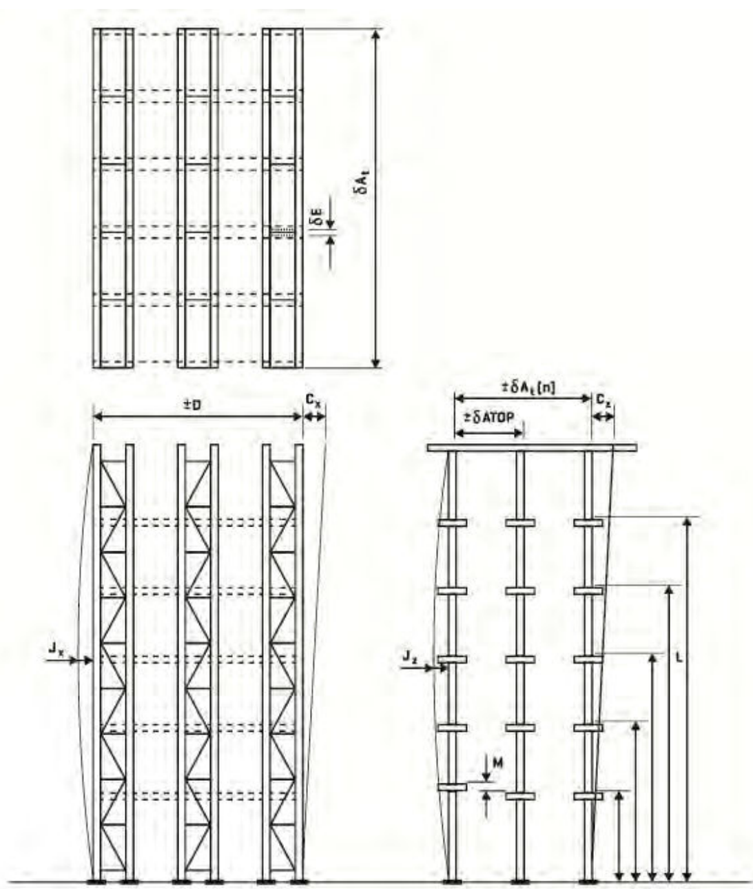
Tolerancias en montaje
