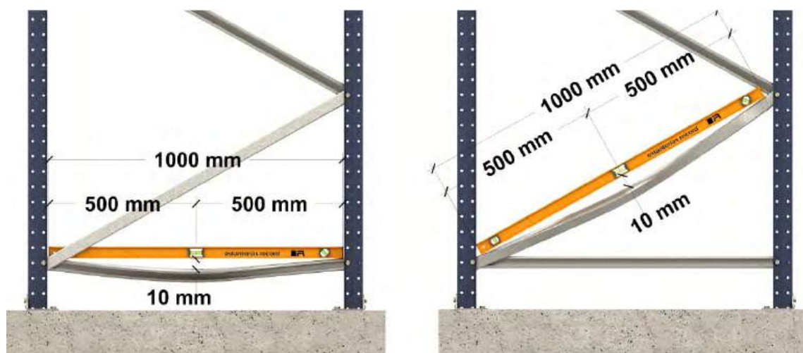
Evaluación de daños en celosías
