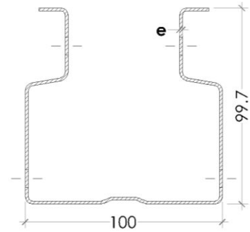
Planta Puntal 100 100
