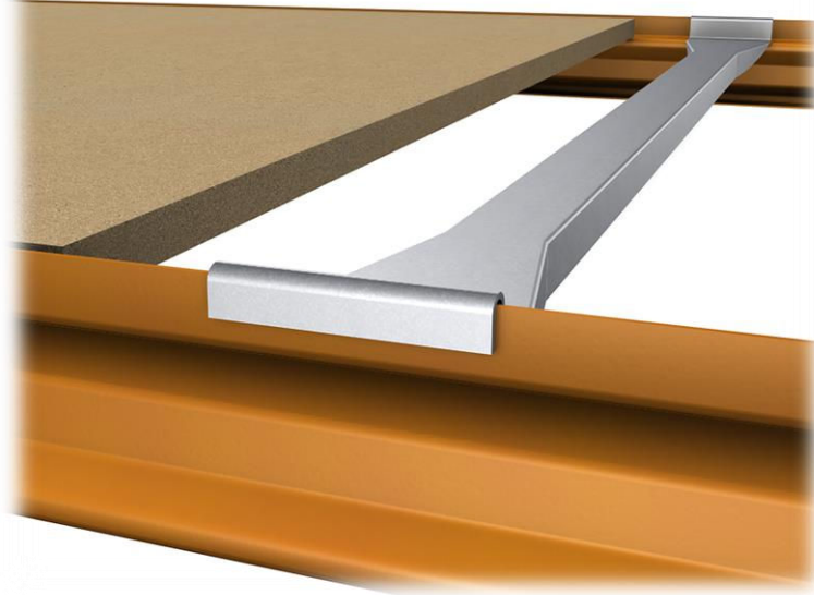
Detalle nivel Picking Z-80 con soportes y aglomerado
