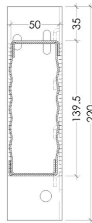
Perfil A-A Larg.140x50
