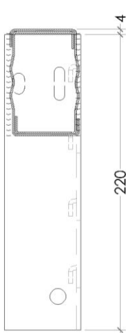
Perfil A-A Larg.80x50
