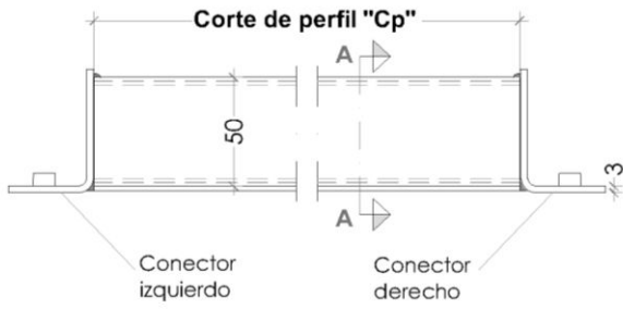
Planta largueros 80, 100, 120,140x50
