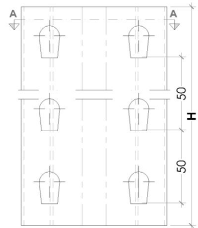
Planta Puntal 100 100
