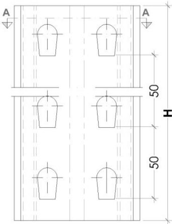
Planta Puntal 80 63
