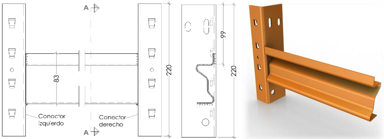
Sección A-A
