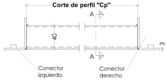
Planta largueros 100, 120x40
