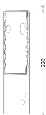
Perfil A-A Larg.140x50
