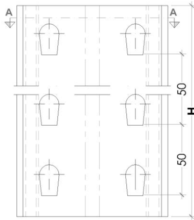
Planta Puntal 100 63
