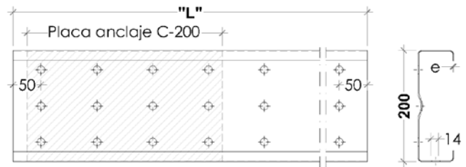
Tracé et profilé base simple 200
