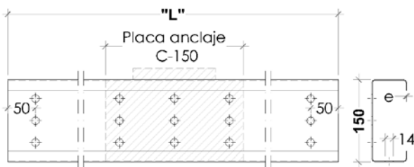
Tracé et profilé base double 150
