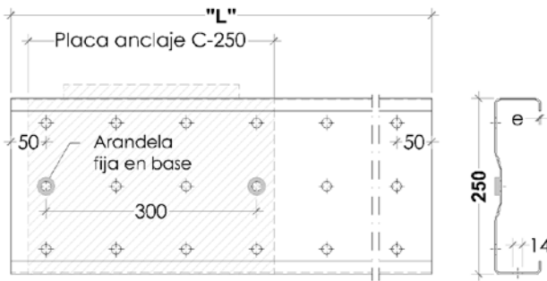
Tracé et profilé base simple 250
