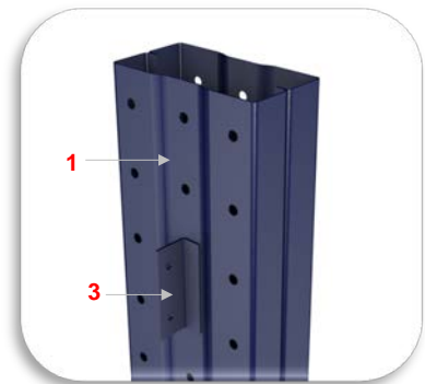
Détail supérieur colonne
