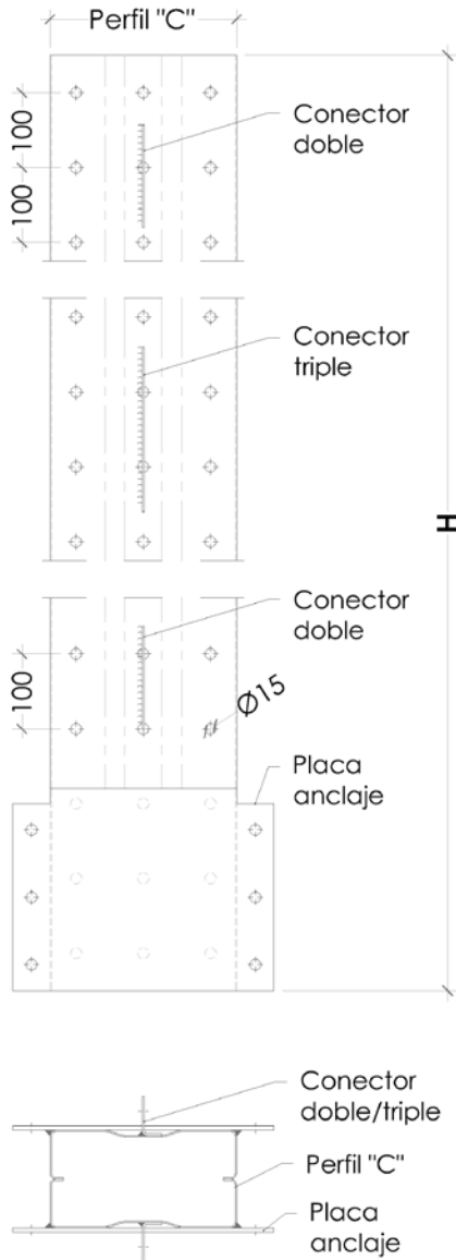
Vue en plan et tracé générique colonne
