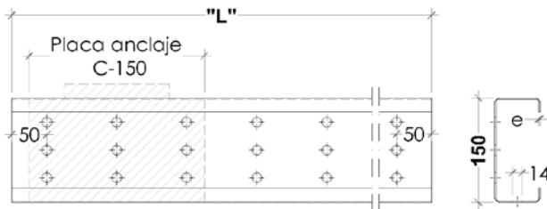
Tracé et profilé base simple 150
