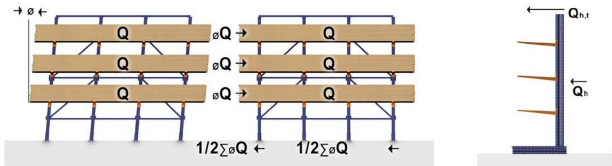
Stabilité longitudinale
