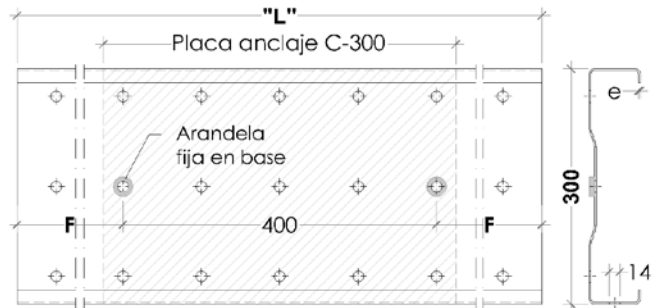
Tracé et profilé base double 300
