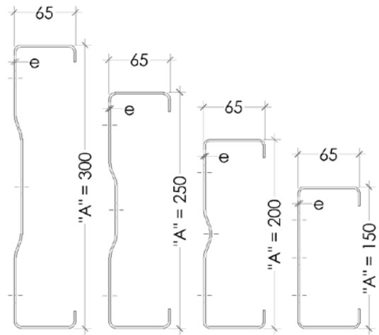
Section A-A profilés « C » e = 2, 2,5, 3 ou 4 mm
