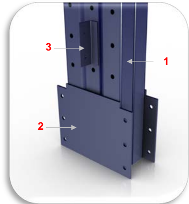
Détail inférieur colonne
