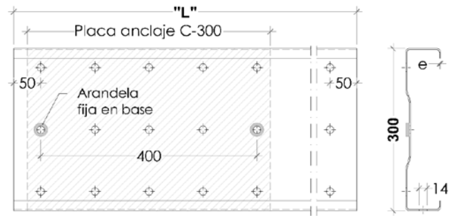
Tracé et profilé base simple 300
