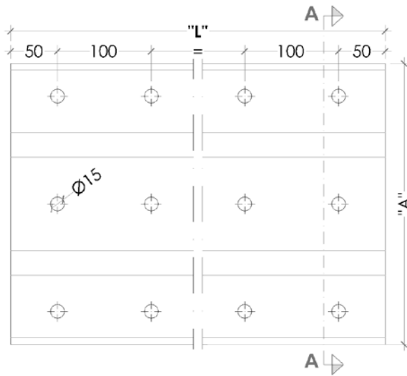
Tracé générique profilé « C » L = coupe de profil
