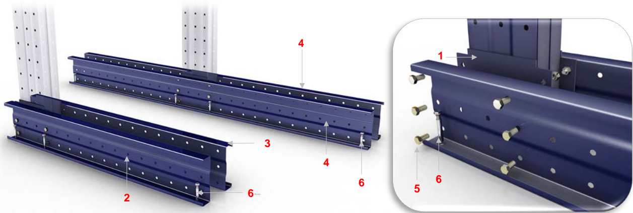
Schéma bases simples, doubles et détail de fixation à colonne
