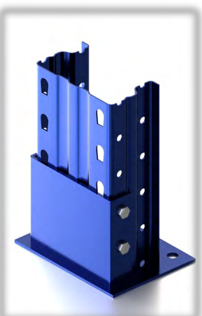
Puntal 100 100 con placa base
