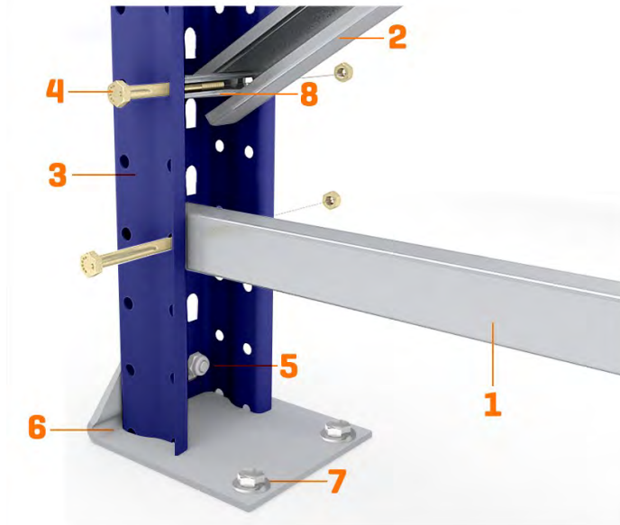
Detalle elementos arriostrados
