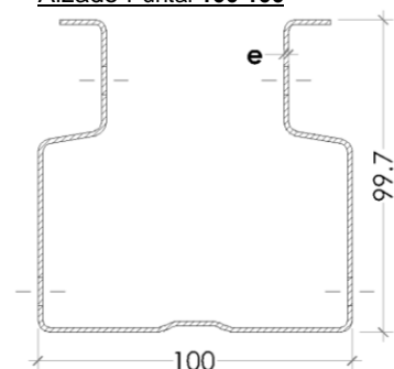
Alzado Puntal 100 100
