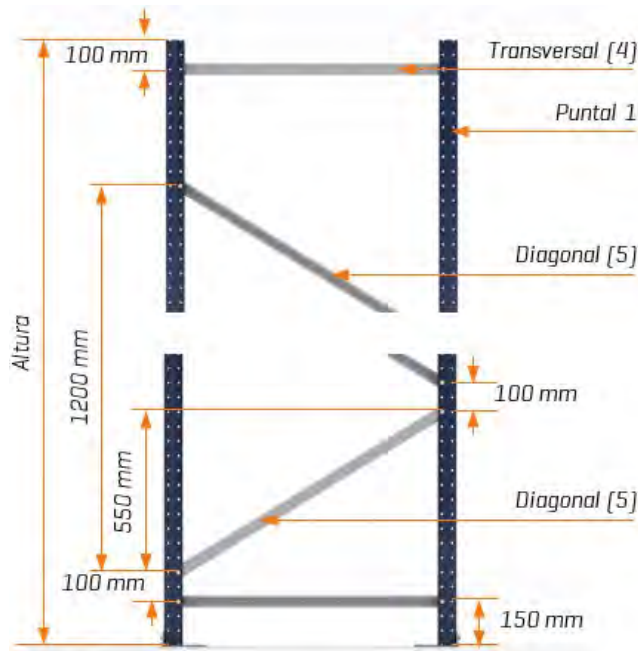
Esquema de montaje tipo 1
