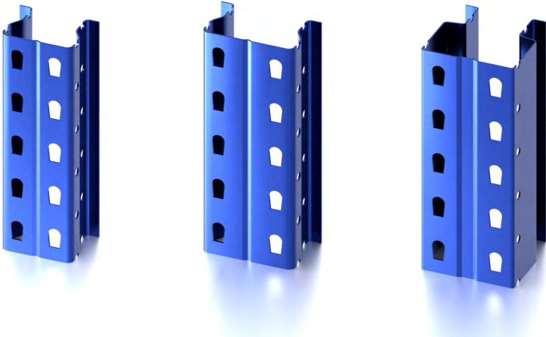
Detalle puntal 80 63, 100 63 y 100 100
