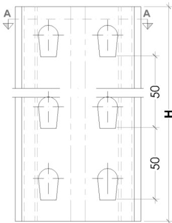
Alzado Puntal 80 63
