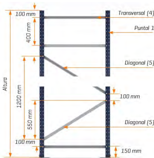
Esquema de montaje tipo 2
