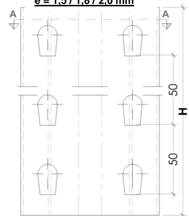
Planta Puntal 100 100 e = 1,5 / 1,8 / 2,0 mm
