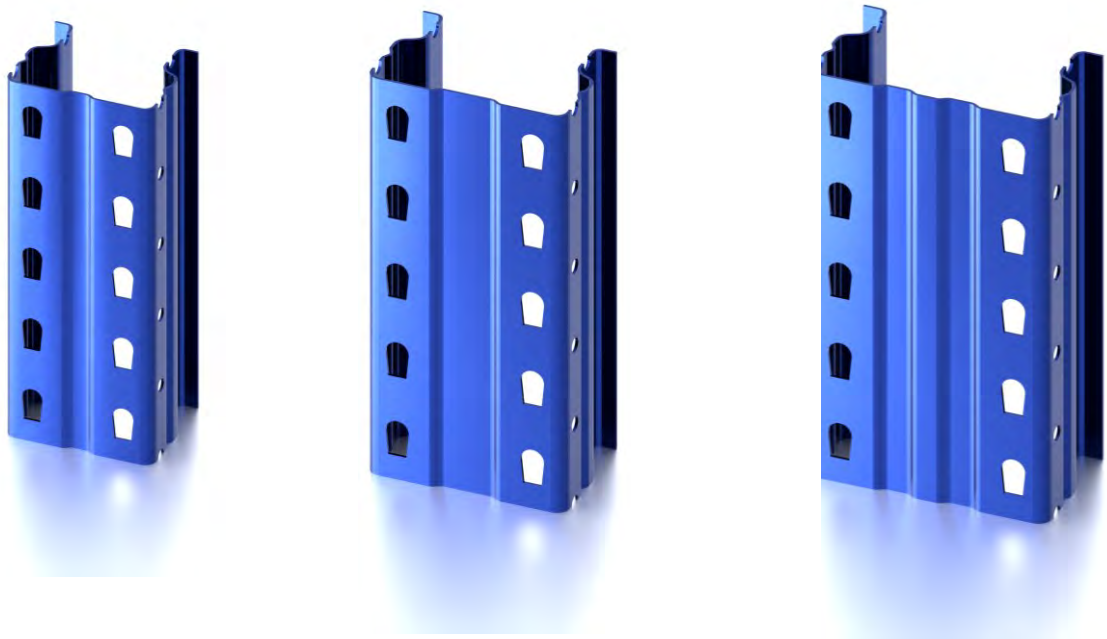
Detalle puntal 100 80, 120 80 y 140 80
