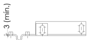
Planta ménsula 80 izquierda.
