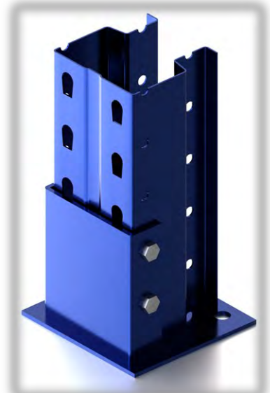
Puntal 100 100 con placa base
