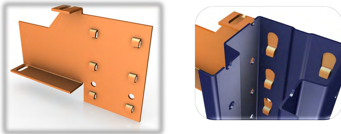
Encastre de ménsulas. Detalle de salientes y posicionamiento en el puntal
