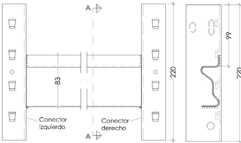
Alzado
