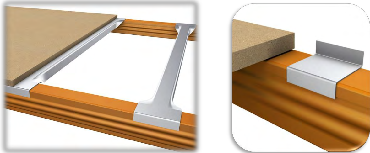
Detalle nivel Picking convencional con soporte y tope retenedor
