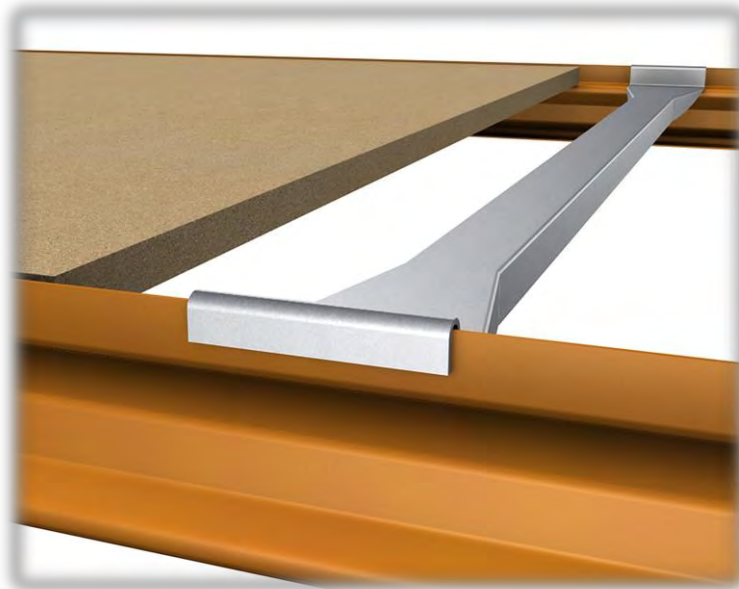
Detalle nivel Picking Z-80 con soportes y aglomerado
