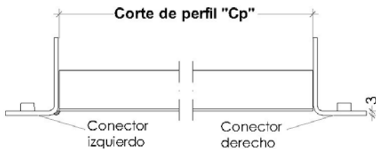
Planta
