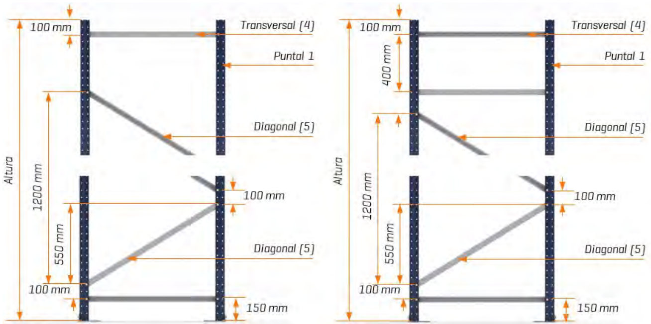
Esquema de montaje tipo 1
