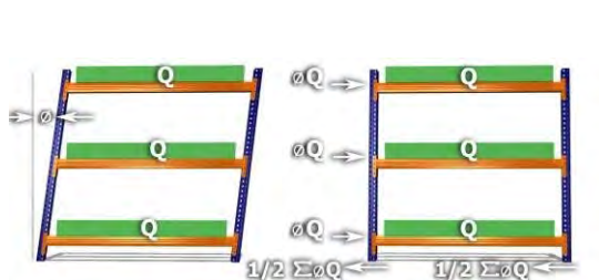
Estabilidad longitudinal
