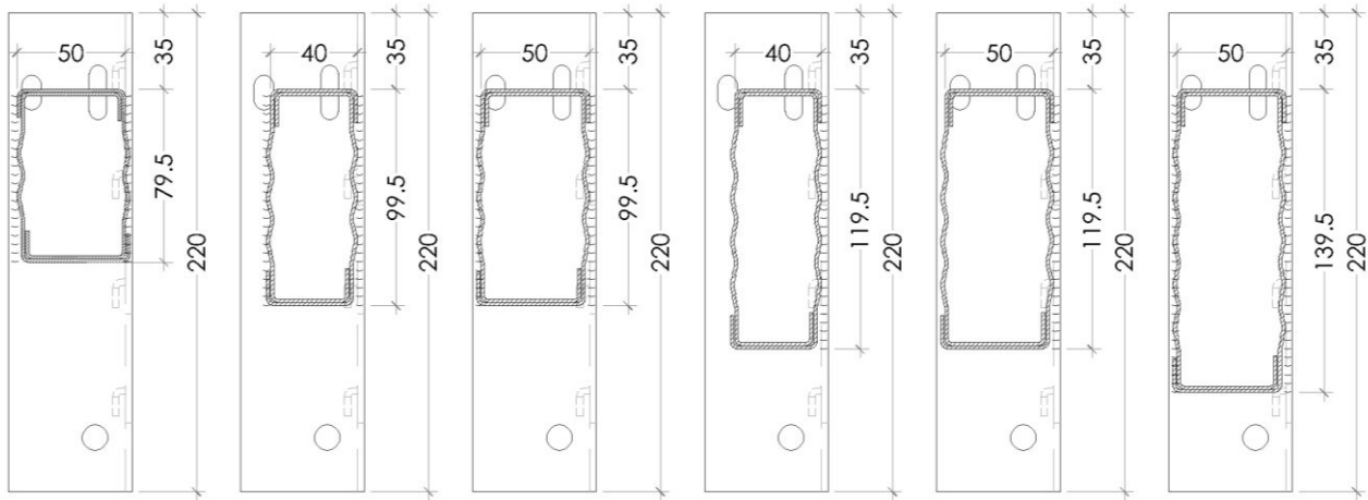
Perfil A-A Larg. 80x50
