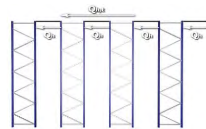
Estabilidad transversal
