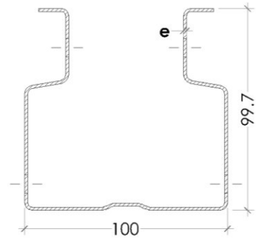
Planta Puntal 100 100
