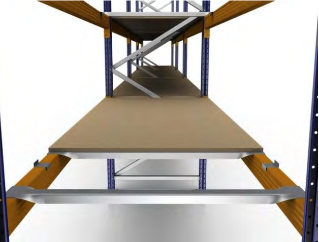
Nivel Picking convencional 80
