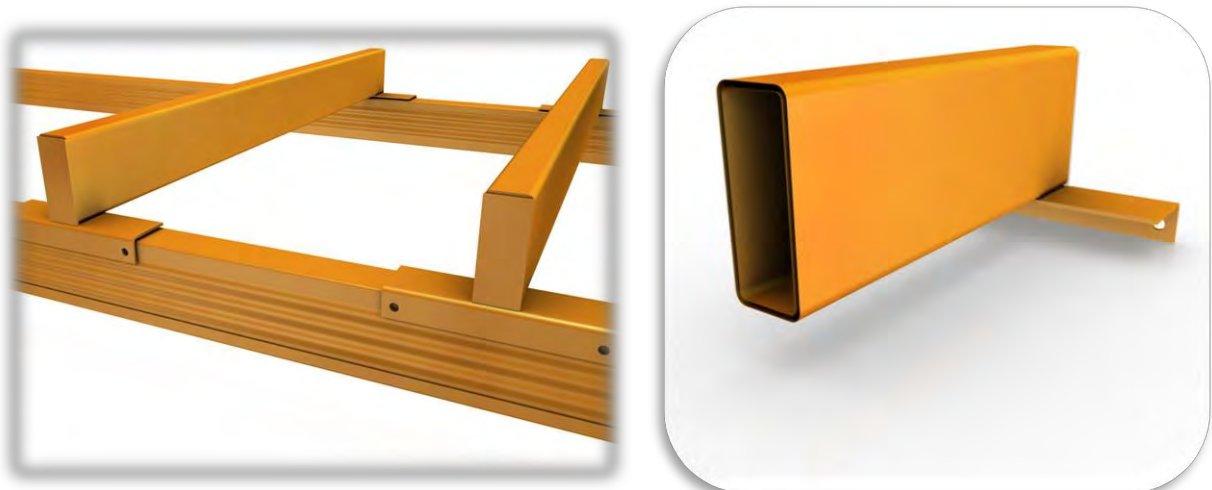
Soporte de paleta elevado. Detalle de posicionamiento y sección transversal
