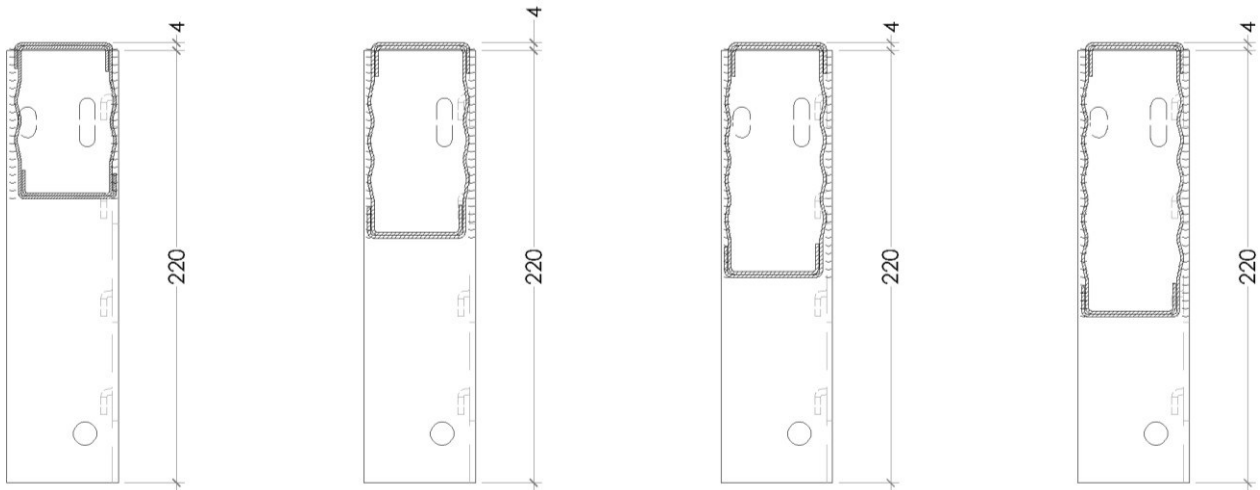
Perfil A-A Perfil A-A Perfil A-A Perfil A-A Larg.80x50 Larg.100x50 Larg.120x50 Larg.140x50
