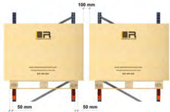
Holguras horizontales en fondo Alineaciones dobles. Paletas con carga saliente
