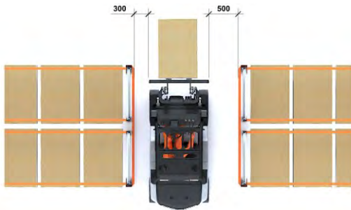
Holguras en pasillos de maniobra Circulación con personal, según UNE-EN 15629
