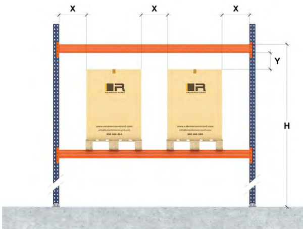
Holguras horizontales y verticales en alveolo Paletas sin carga saliente situadas en niveles elevados
