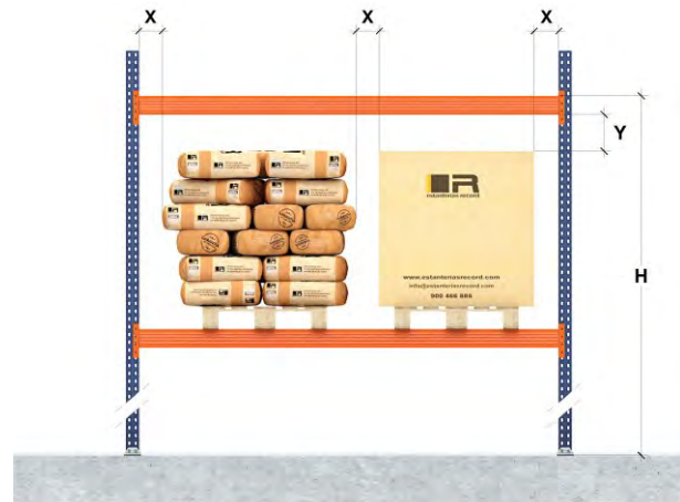
Holguras horizontales y verticales en alveolo Paletas con carga saliente situadas en niveles elevados
