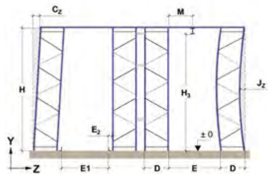
Esquema vista lateral Clase 300
