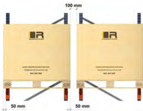
Holguras horizontales en fondo Alineaciones dobles. Paletas con carga sin saliente
