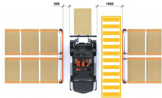
Holguras en pasillos de maniobra Circulación con personal, según NTP 852
