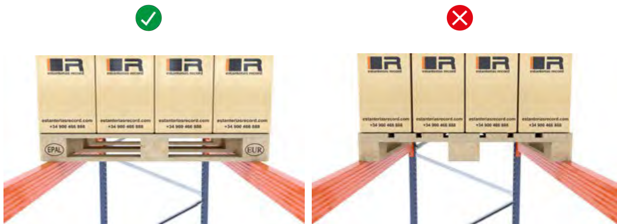
Posicionamiento de la paleta sobre los largueros
