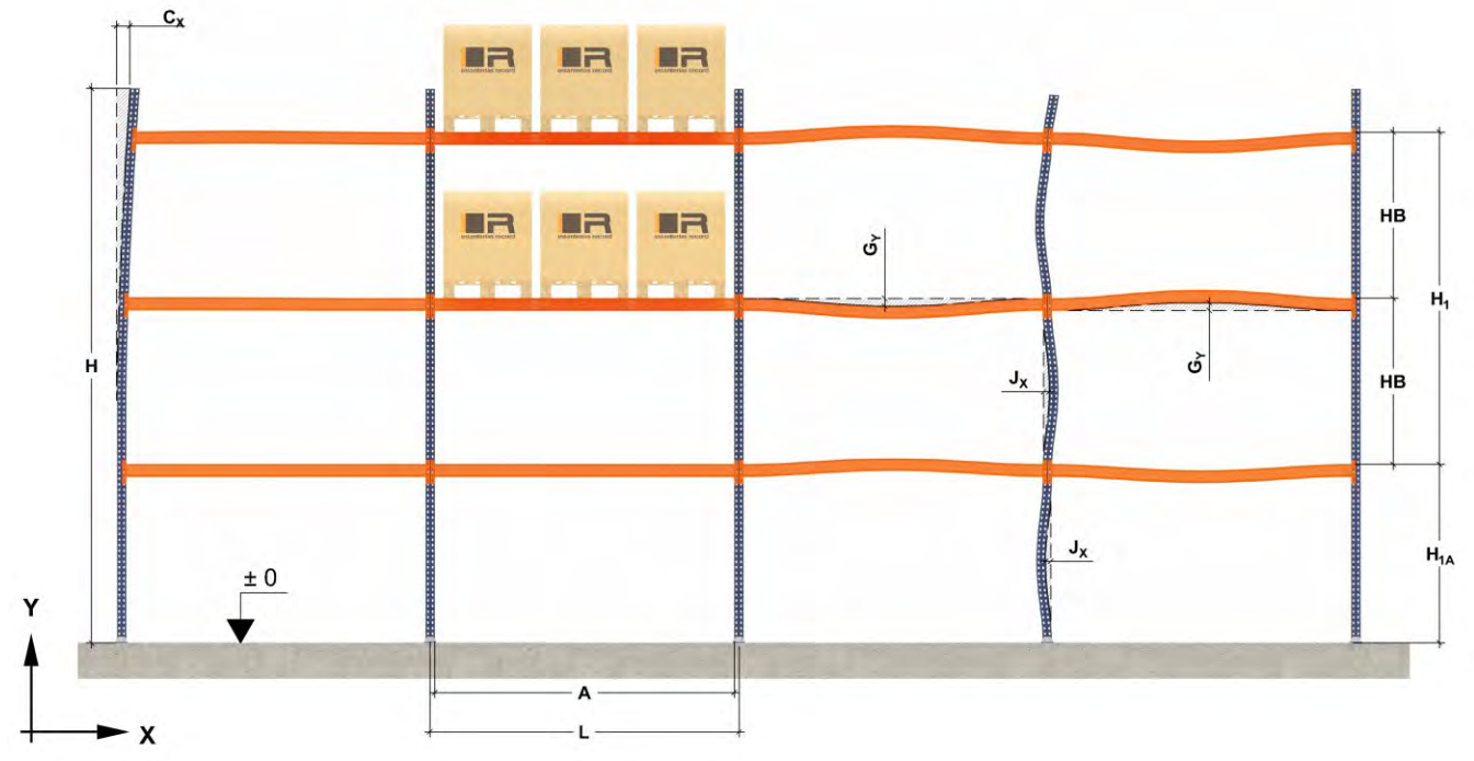
Esquema vista frontal Clase 400 y Clase 300
