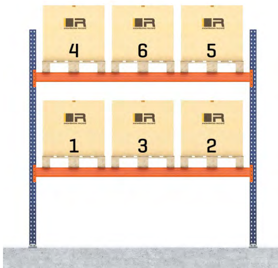
Secuencia correcta de carga
