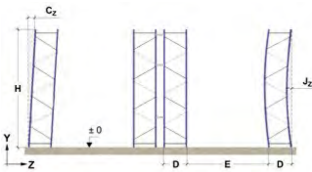
Esquema vista lateral Clase 400
