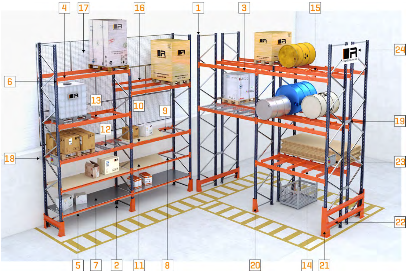
Esquema genérico de paletización convencional, componentes y accesorios.
