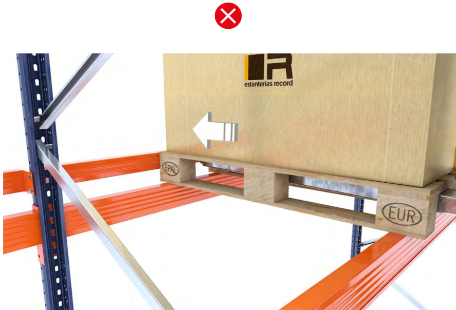
Sobrecarga producida por empuje o impacto en el larguero tope paleta
