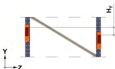
Desalineación de los largueros del nivel de carga
