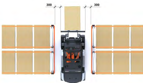
Holguras pasillo de maniobra, circulación simple
