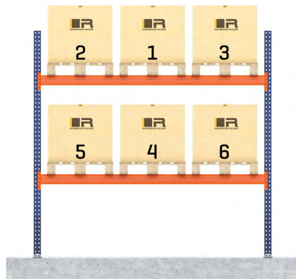
Secuencia correcta de descarga
