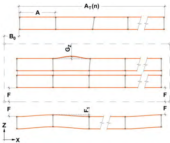
Esquema vista superior Clase 400
