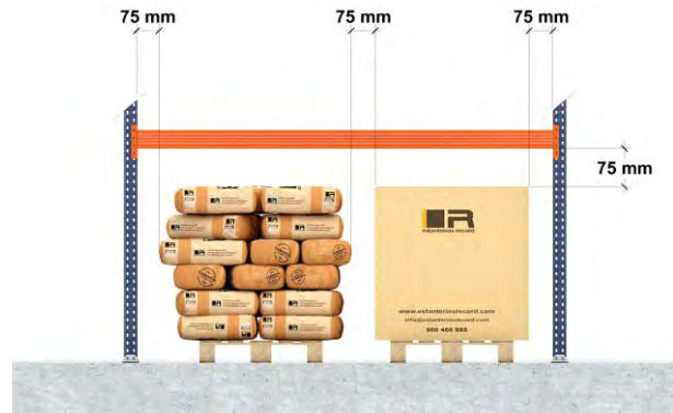
Holguras horizontales y verticales en alveolo Paletas con carga saliente situadas en el suelo
