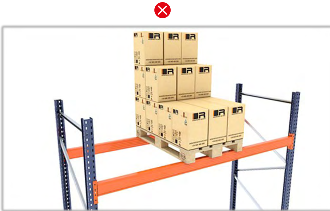
Sobrecargas por asimetría de carga en la paleta
