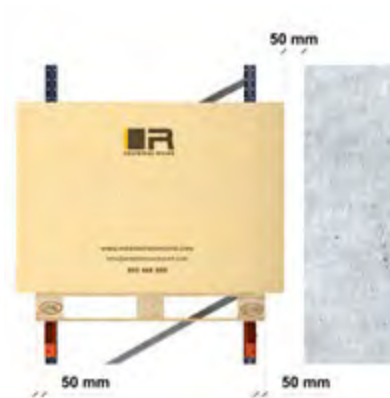
Holguras horizontales en fondo Alineaciones simples. Paletas con carga saliente
