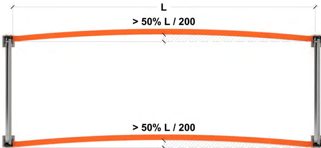
Deformación residual horizontal [sin carga] superior al 50 % de la flecha nominal vertical [con carga]
