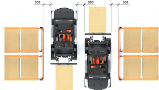
Holguras pasillo de maniobra, circulación doble
