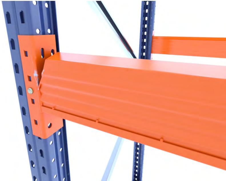
Soldadura de conector-larguero desgarrada
