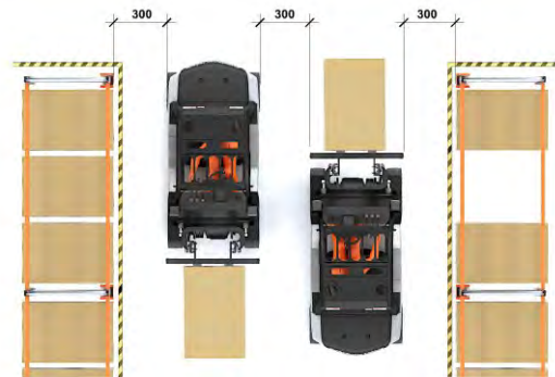
Holguras pasillo de trabajo, circulación doble
