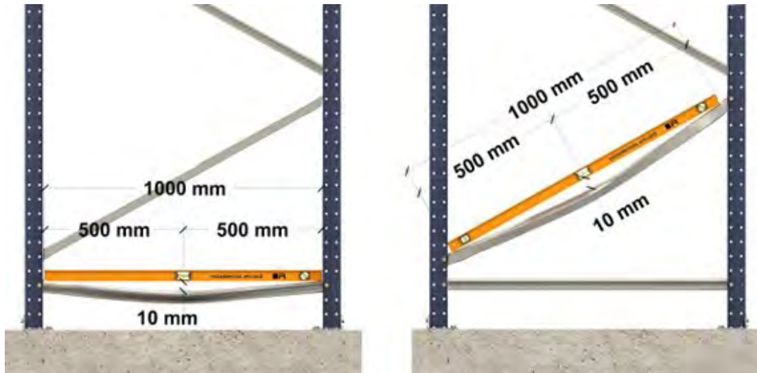
Evaluación de daños en celosías
