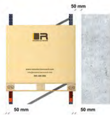
Holguras horizontales en fondo Alineaciones simples. Paletas con carga sin saliente
