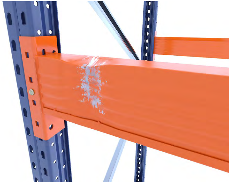
Larguero dañado por abolladura
