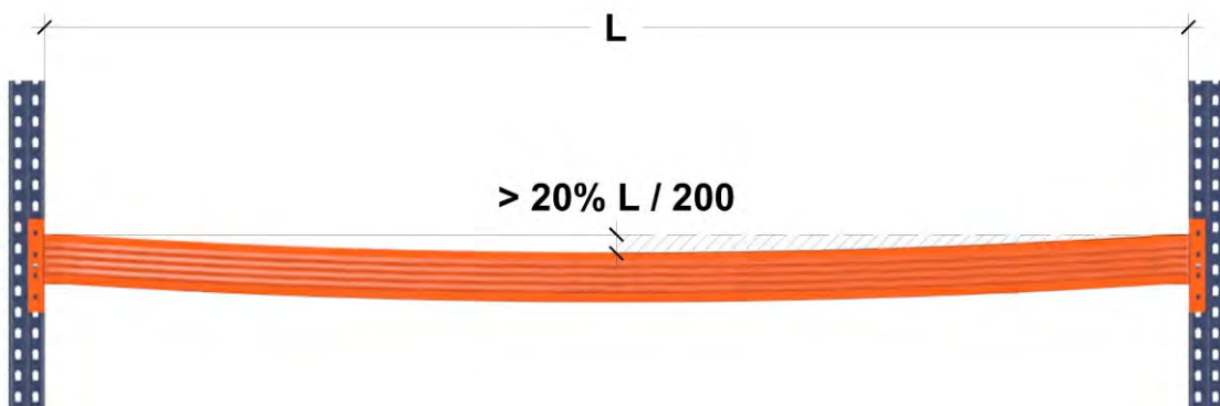
Deformación residual vertical [sin carga] superior al 20 % de la flecha nominal vertical [con carga]
