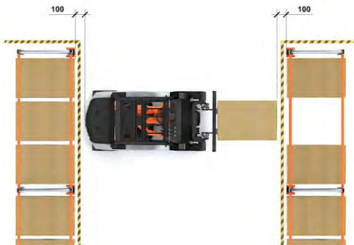
Holguras pasillo de trabajo, circulación simple
